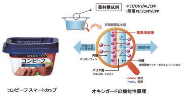
図2 多層ハイバリア構成による金属代替のスマートカップとオキシガードの原理 4)
