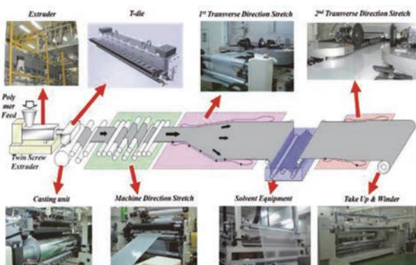
図 12 セパレータ製造ラインの装置構成
