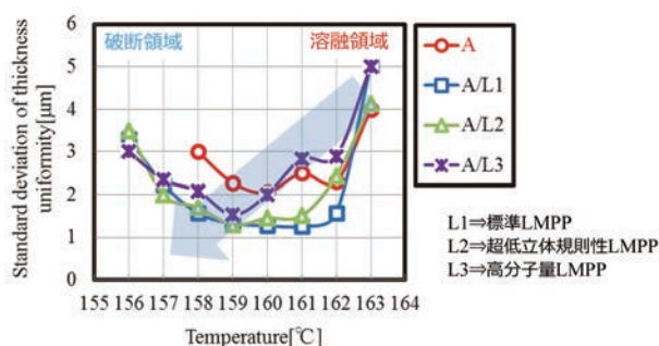
図9 延伸可能温度幅と偏肉精度
