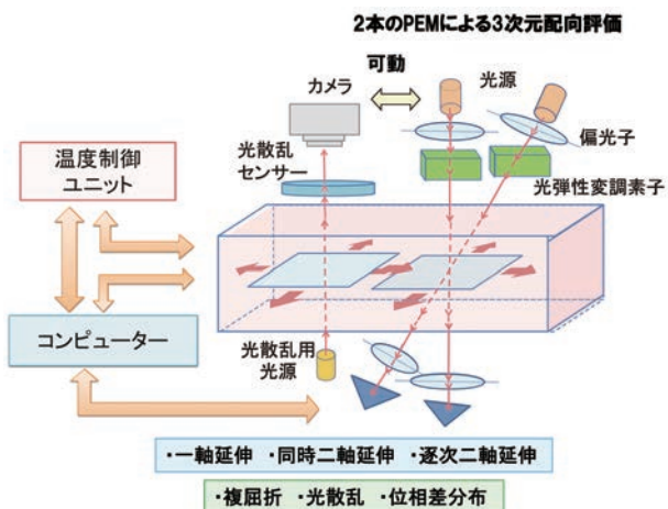
図8 二軸延伸フィルム試験機
