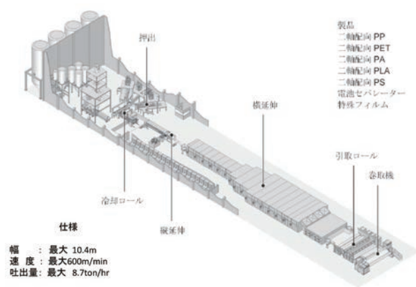
図7 逐次二軸延伸ライン
