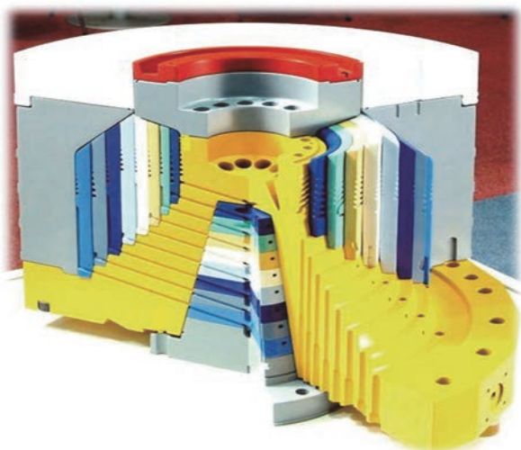
図3 9層のスパイラルダイスの構造
