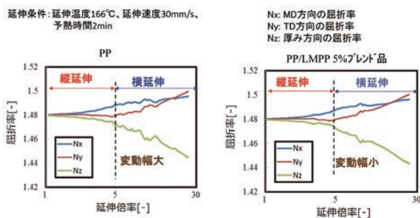
図10 3次元屈折率(超低立体規則性PP添加有無の比較)
