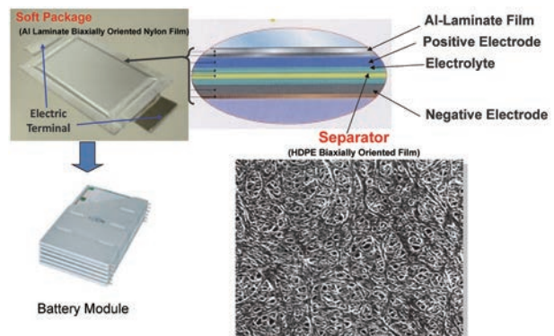
図 13 Li-ion Battery (セパレーター, ソフトパッケージ)
