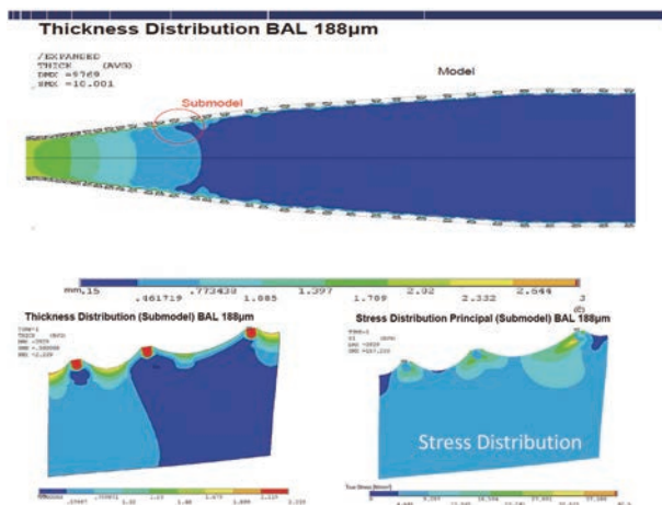
図 11 同時二軸延伸中の厚みと応力解析例
