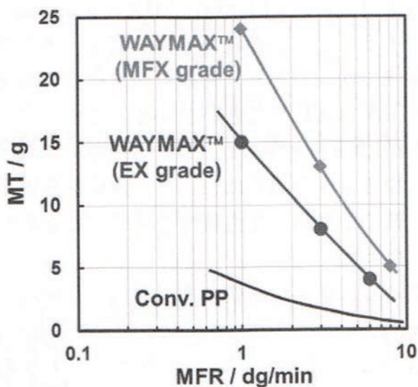
図5 高熔融張力PP(WAYMAX)と一般PPのMFR-MTの比較
